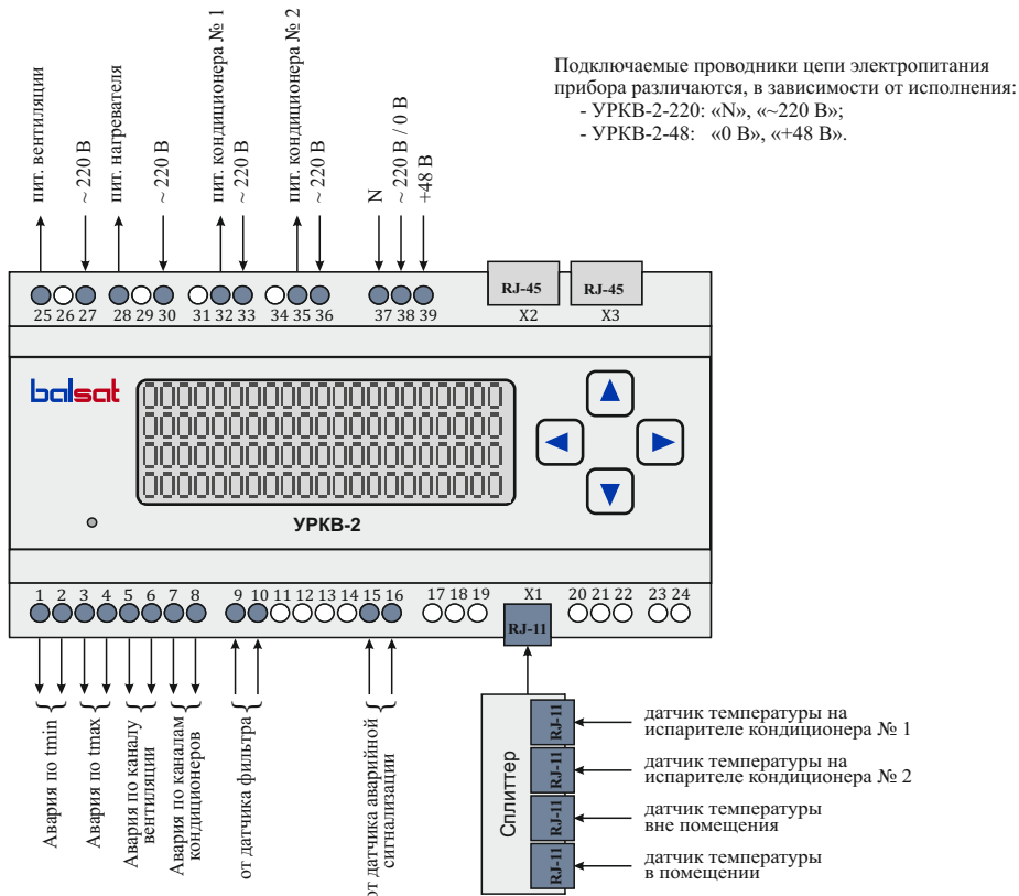
Рисунок 2 - Схема подключения УРКВ-2
